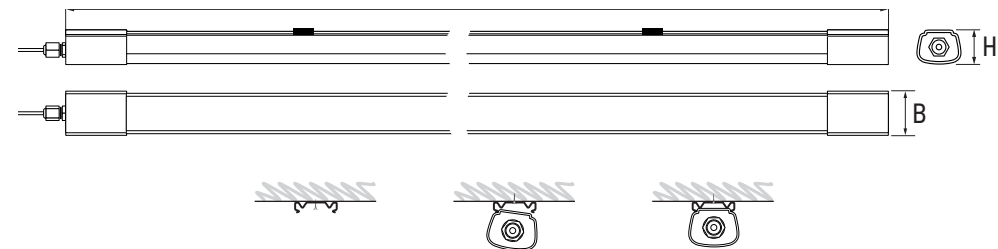
Рис.2 Схема монтажа светильника
